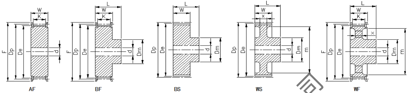
H型标准皮带宽100 (25.4mm)
