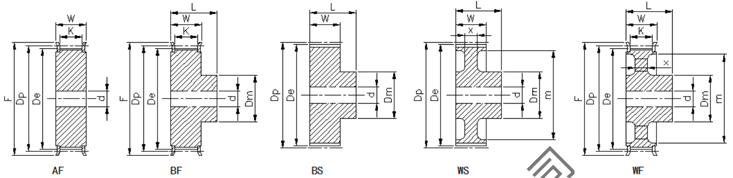
XL型标准皮带宽037 (9.5mm)
