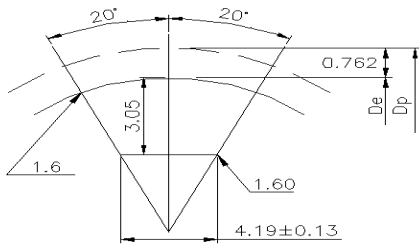
H型齿形图:
