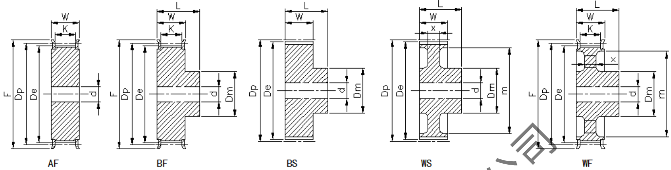
XH型标准皮带宽300 (76.2mm)
