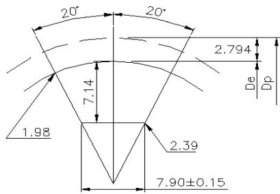
XH型齿形图:
