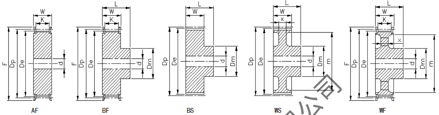
XL型标准皮带宽050 (12.7mm)
