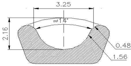
5M型齿形图:
