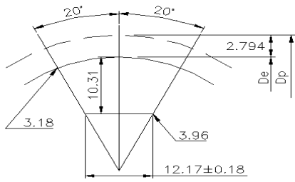
XXH型齿形图:
