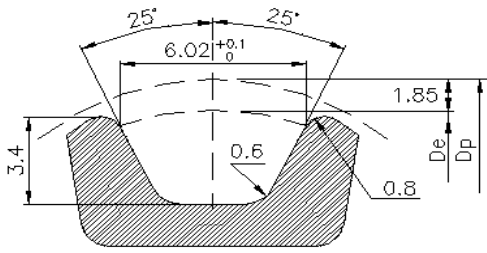
T10型齿形图:
