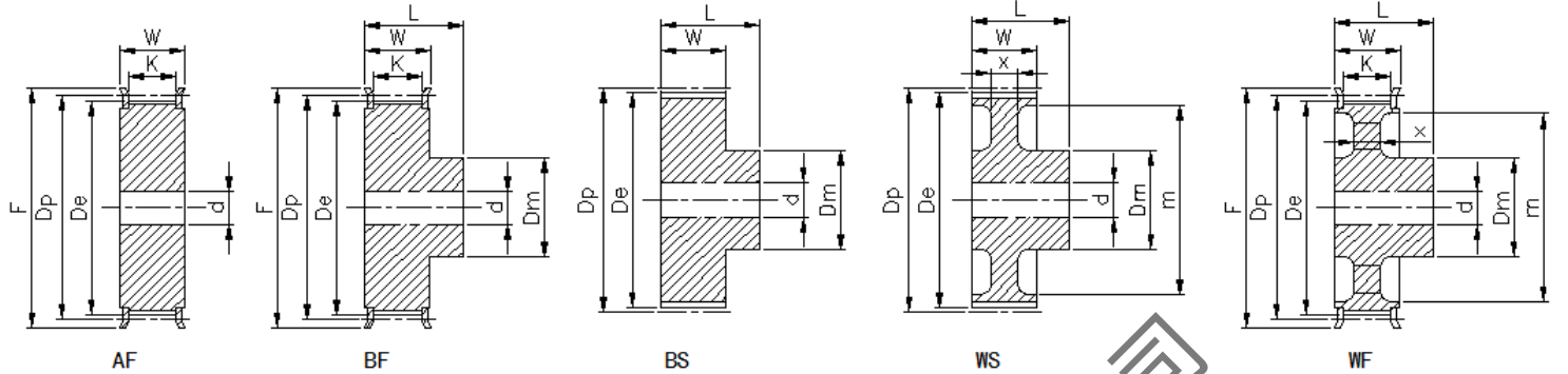
T20型标准皮带宽 (100mm)
