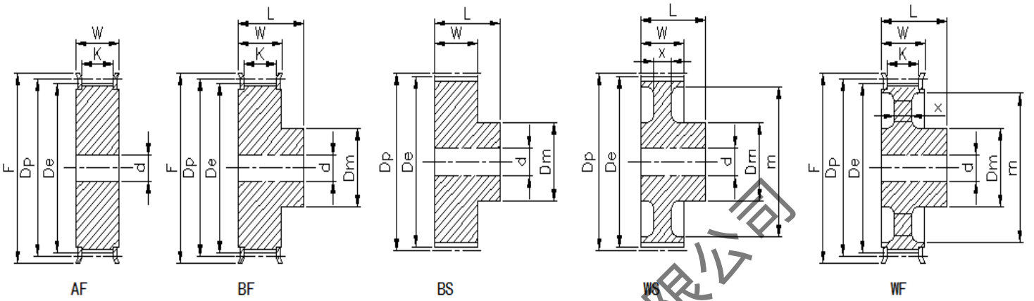
T10型标准皮带宽 (30mm)
