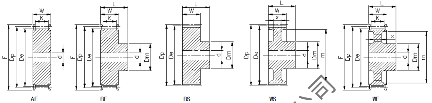
XH型标准皮带宽200 (50.8mm)
