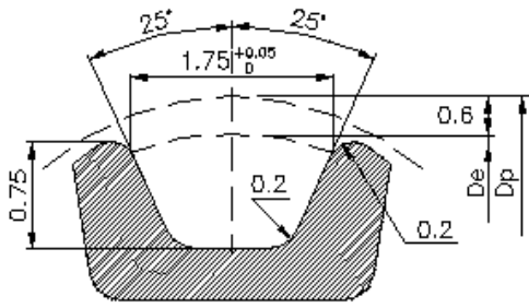
T2.5型齿形图:
