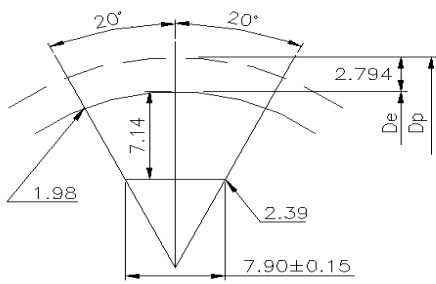
XH型齿形图:
