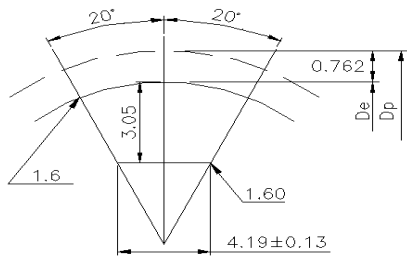
H型齿形图:
