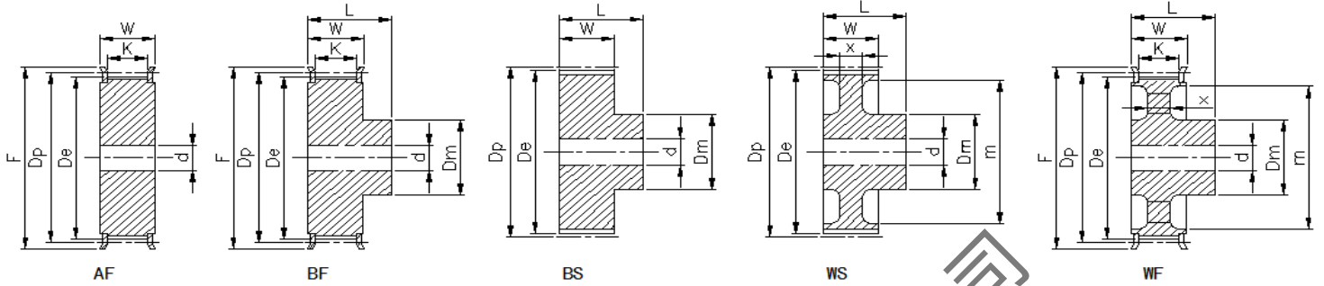
L型标准皮带宽075 (19.1mm)
