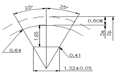
XL型齿形图:
