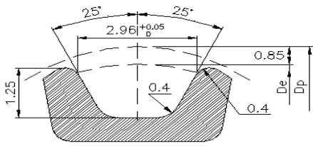
T5型齿形图:
