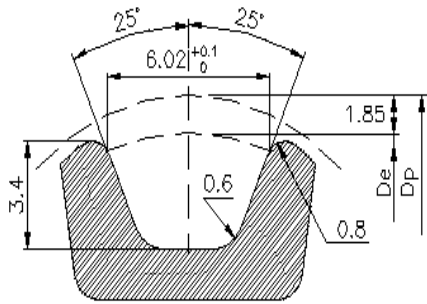
T10型齿形图:
