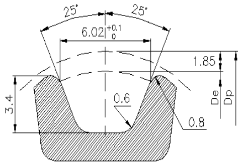
T10型齿形图:
