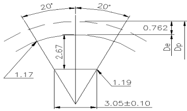
L型齿形图:
