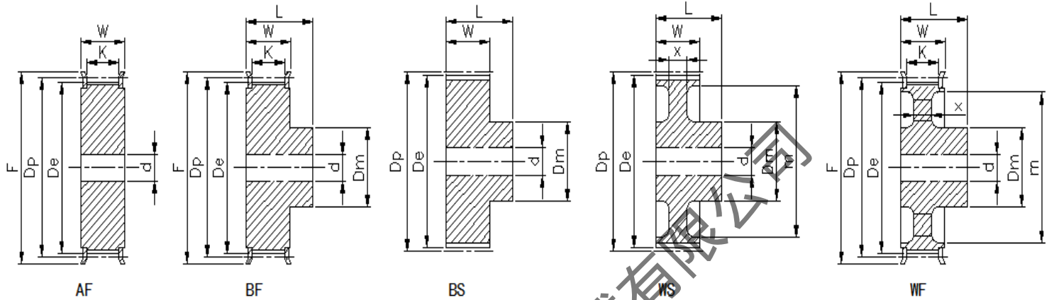
T10型标准皮带宽 (50mm)
