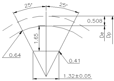
XL型齿形图:
