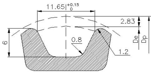
T20型齿形图:
