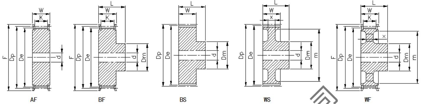
H型标准皮带宽150 (38.1mm)
