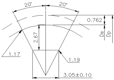
L型齿形图:
