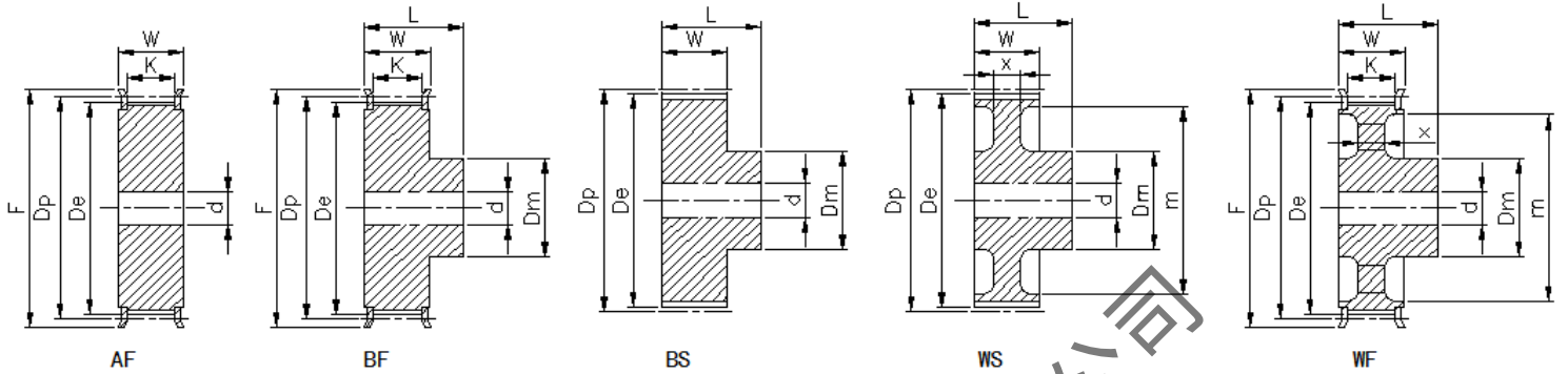
T20型标准皮带宽 (50mm)
