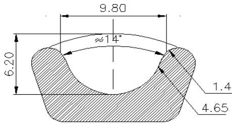
14M型齿形图:
